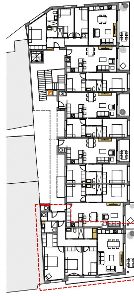
HABITATGE 1A - PLANTA PRIMERA
