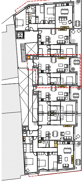
HABITATGE 2D - PLANTA SEGONA
