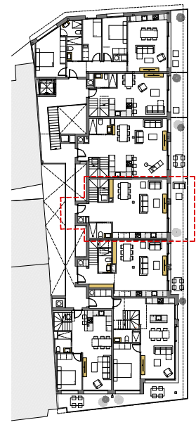
HABITATGE 3D - PLANTA TERCERA
